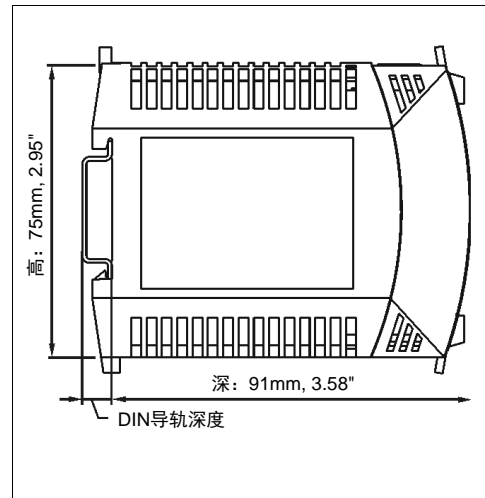
图 22-2 侧视图
