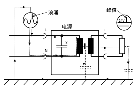
图 24-6 未接地输入
