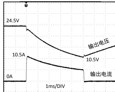
图 24-2 时长 5ms 的 5 倍额定电流的峰值负载，典型值
