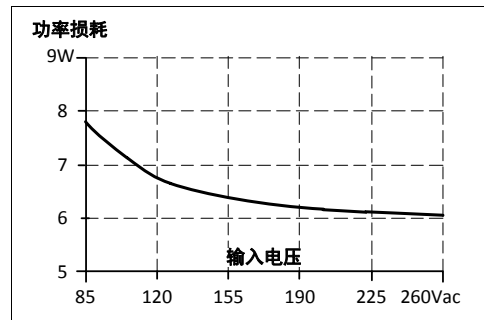
图 8-4 24V/2.1A 时的损耗和输入电压, 典型值
