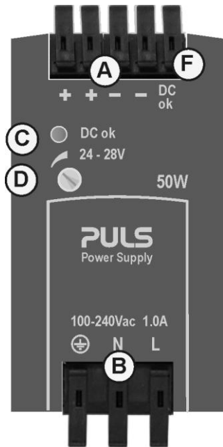
图 10-1 前面板
