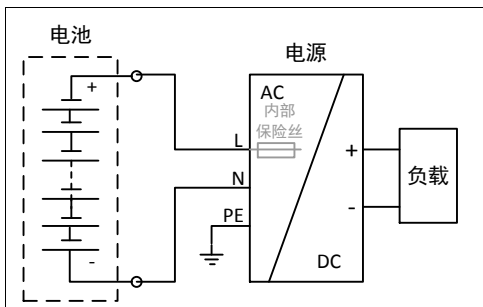
图 7-1 直流输入接线
