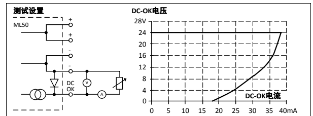
图 12-2 DC-OK 信号输出特性
