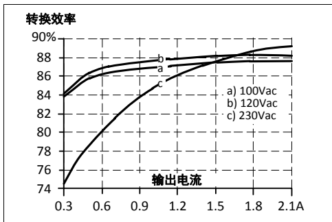
图 8-1 24V 时的转换效率与输出电流, 典型值
