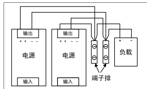
图 24-4 使用端子排
