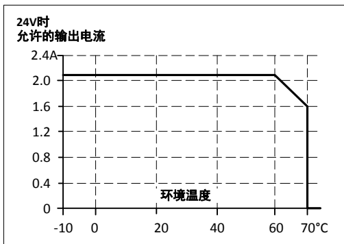
图 15-1 输出功率与环境温度
