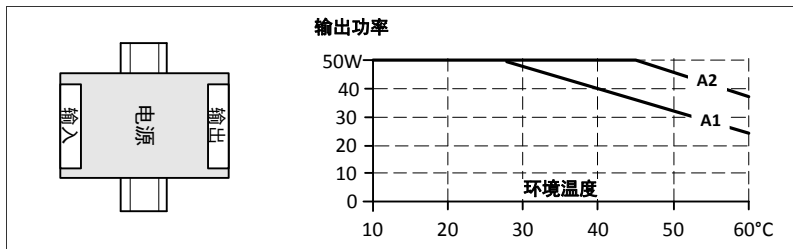
图 24-10 安装方向 D (顺时针平置)
