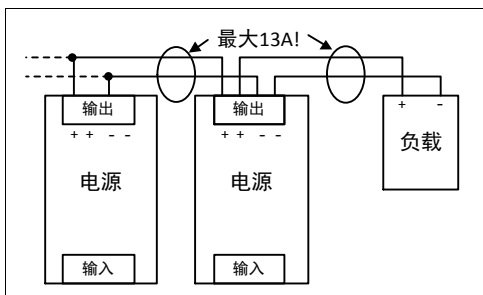
图 24-3 输出的级联式连接
