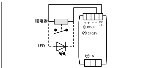
图 12-1 DC-OK 布线图
