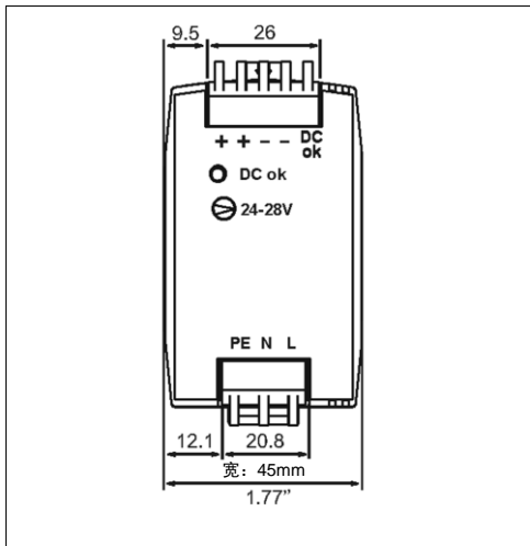
图 22-1 正面图
