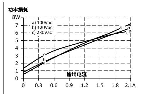
图 8-2 24V 时的损耗与输出电流, 典型值
