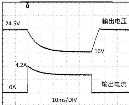
图 24-1 时长 50ms 的 2 倍额定电流的峰值负载，典型值
