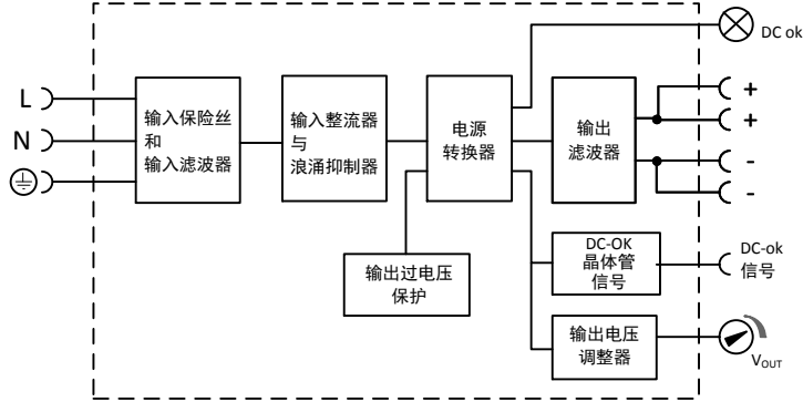
图 9-1 功能图
