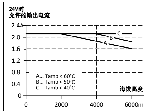
图 15-2 输出功率与海拔高度
