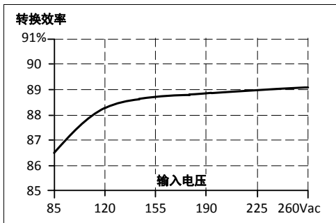
图 8-3 24V/2.1A 时的转换效率与输入电压, 典型值
