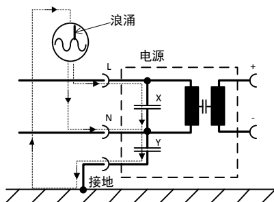
图 24-5 已接地输入
