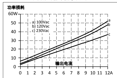
图 9-2 48V 时的损耗与输出电流, 典型值
