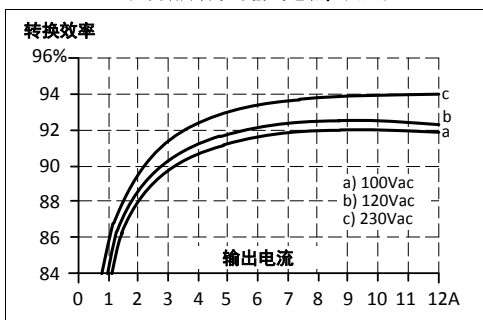
图 9-1 48V 时的转换效率与输出电流, 典型值
