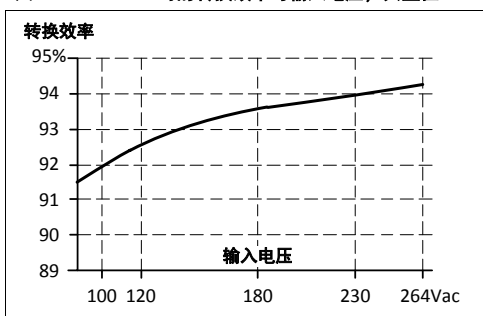
图 9-3 48V/10A 时的转换效率与输入电压, 典型值
