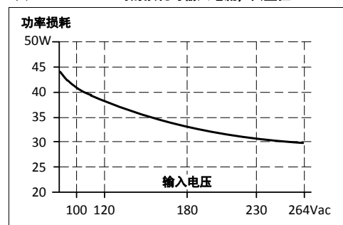
图 9-4 48V/10A 时的损耗与输入电压, 典型值
