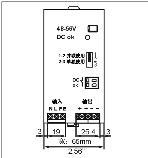
图 20-1 正面图
