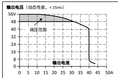
图 6-4 动态过电流能力，典型值
