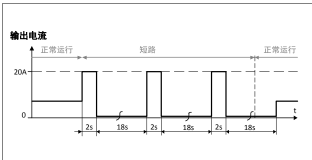
图 6-3 输出短路，Hiccup PLUS 打嗝模式，典型值
