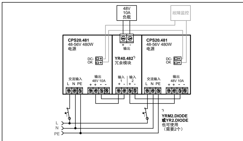
图 21-1 配备双通道冗余模块的 48V/10A 典型 1+1 冗余配置
