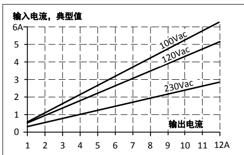
图 3-3 48V 时的输入电流与输出负载
