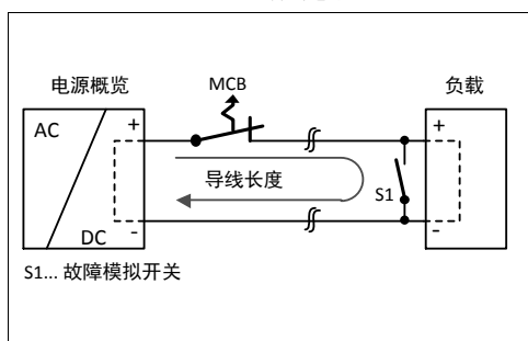
图 22-3 测试电路
