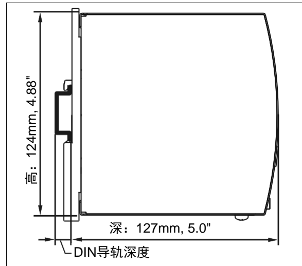
图 20-2 侧视图
