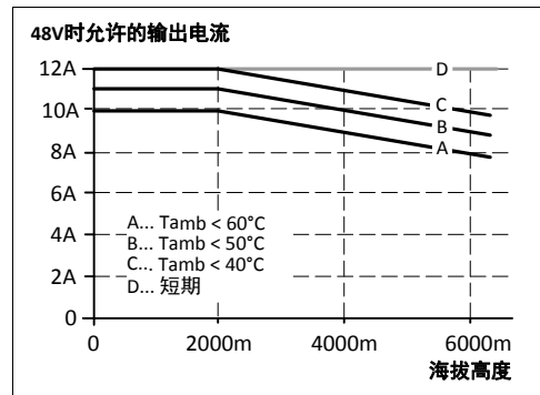
图 15-2 输出电流和海拔高度
