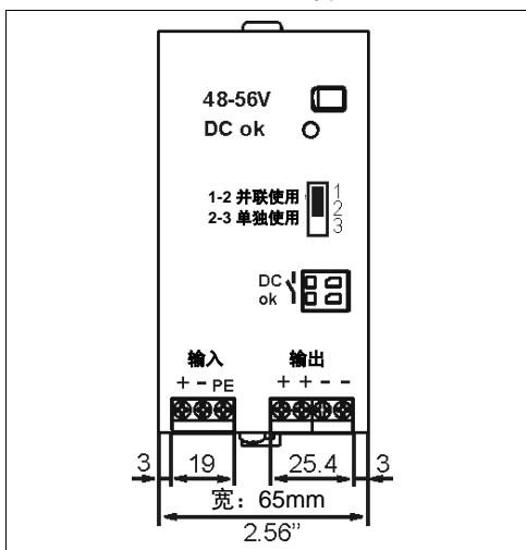
图 20-1 正面图
