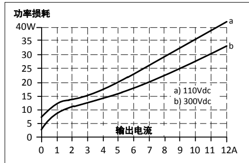
图 9-2 48V 时的损耗与输出电流, 典型值
