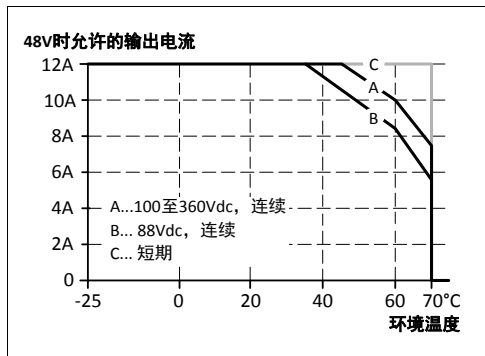
图 15-1 输出电流和环境温度
