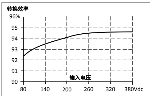
图 9-3 48V/10A 时的转换效率与输入电压, 典型值
