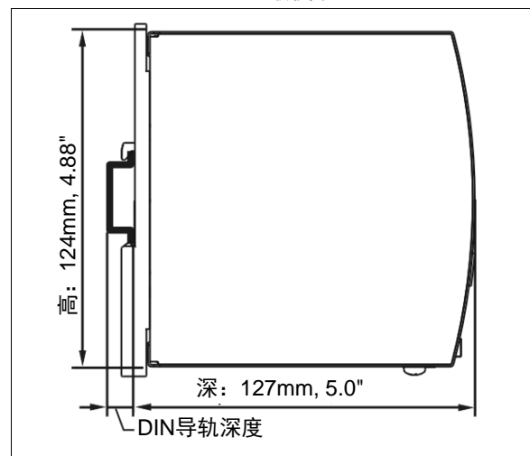
图 20-2 侧视图
