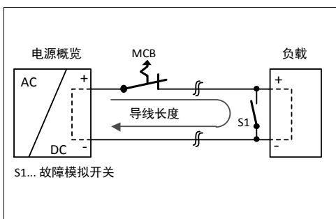
图 22-3 测试电路
