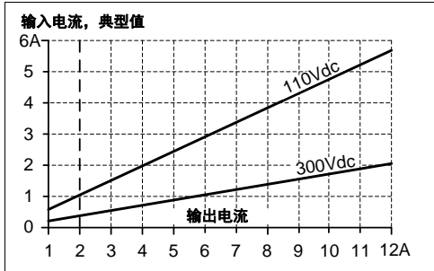
图 4-3 48V 时的输入电流与输出负载
