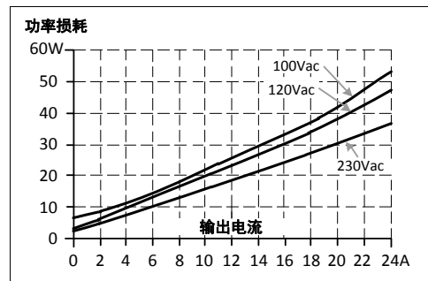
图 9-2 24V 时的损耗与输出电流, 典型值
