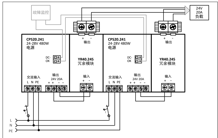
图 21-2 配备多个 YR40.245 冗余模块的 20A 典型 N+1 或 1+1 冗余配置
