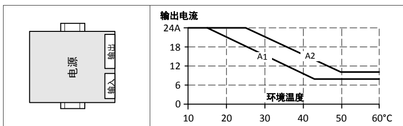
图 22-9 安装方向 E (逆时针平置)
