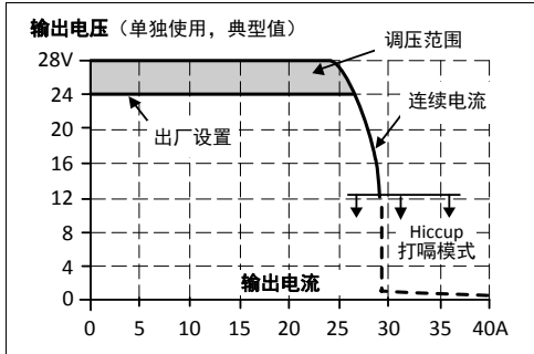
图 6-1 输出电压和输出电流，典型值
