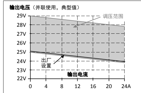
图 6-2 “并联使用”模式下的输出电压，典型值
