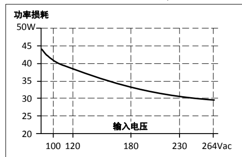
图 9-4 24V/20A 时的损耗与输入电压, 典型值
