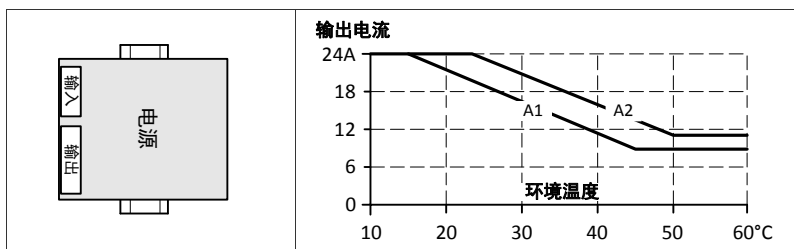
图 22-8 安装方向 D (顺时针平置)
