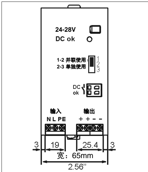
图 20-1 正面图
