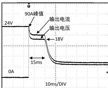
图 22-3 90A 峰值负载，典型值
