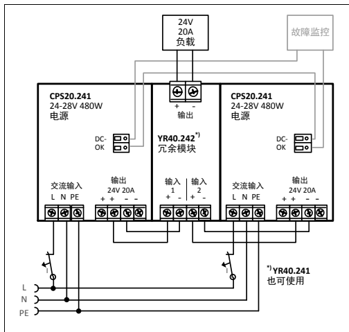
图 21-1 配备双通道冗余模块的 20A 典型 1+1 冗余配置
