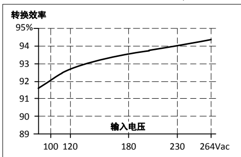
图 9-3 24V/20A 时的转换效率与输入电压, 典型值
