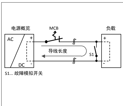
图 22-4 测试电路
