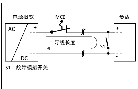
图 22-4 测试电路
