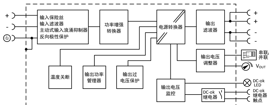
图 11-1 功能图
