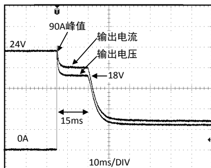
图 22-3 90A 峰值负载，典型值
