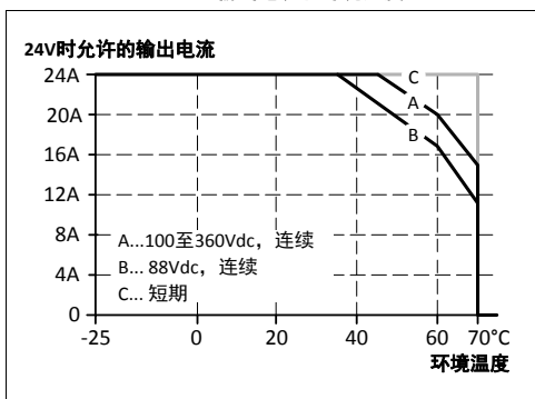
图 15-1 输出电流和环境温度
