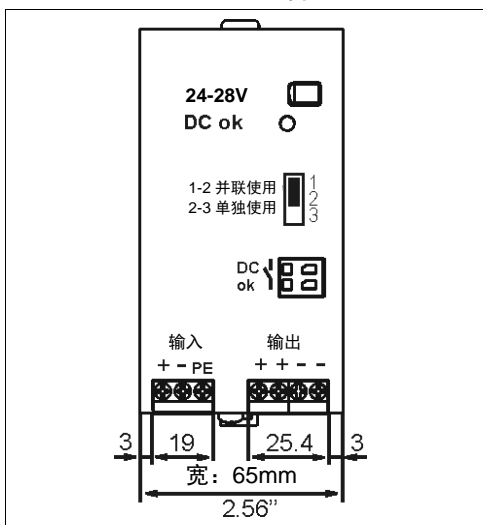
图 20-1 正面图
