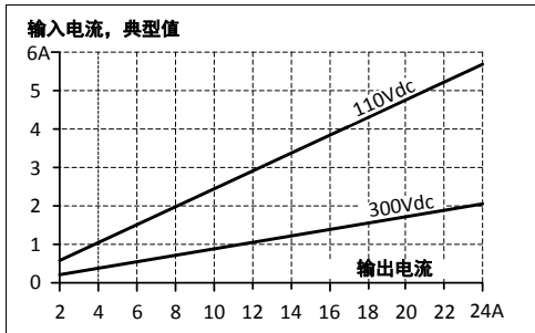
图 4-3 24V 时的输入电流与输出负载
